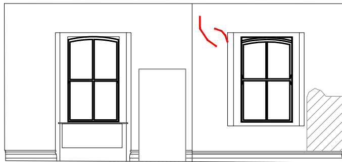
Elevation No 4
